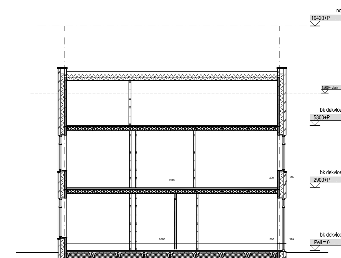
Doorsnede A-A
