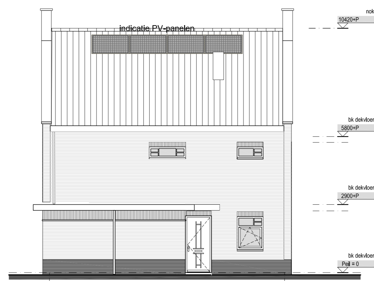
Zijgevel
